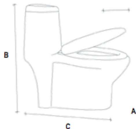
**Dubai Premium 6MWC6 A = 39 cm B = 74.5 cm C = 70 cm Peso: 38 Kg
