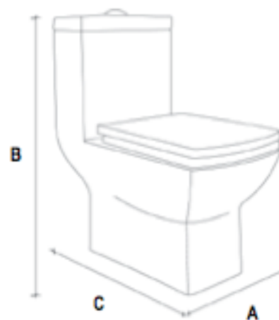
*** Dubai Cuadrato 6MWC14 ***A = 35 cm B = 76 cm C = 63 cm Peso: 40.5 Kg
